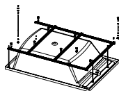
Legset 16 207100
