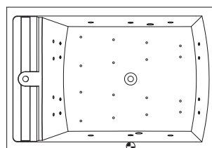
16 aerojets | 6+8+4 hydrojets
